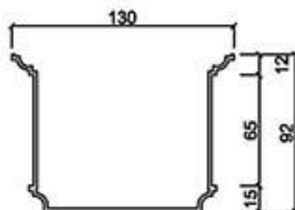
側面圖
