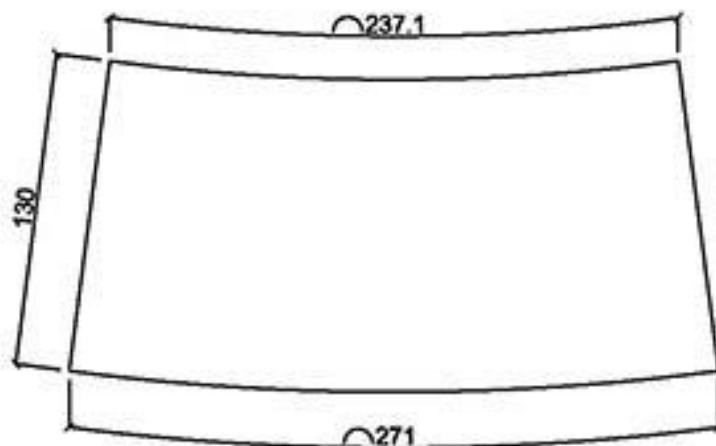
平面圖
