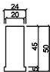
中心剖面圖
